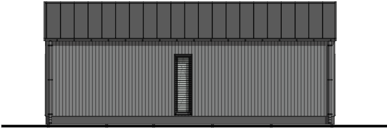
F3 ELEVATION 1:100
