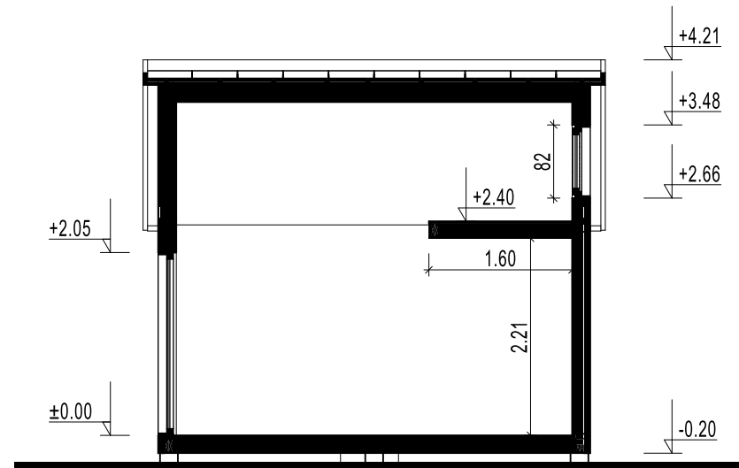
B GRIEZUMS 1:75
